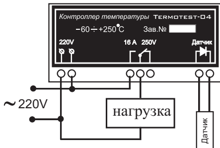
Рис.2 Схема подключения.
