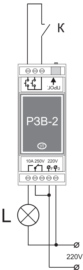
Рис 1. При замыкании контакта К лампа Л включается, после размыкания начинается отсчет времени по истечении которого лампа выключается. В качестве К может быть кнопка без фиксации или обычный выключатель.
