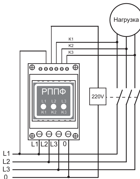
Рис.1 Вариант схемы подключения с контролем контактов пускателя.
