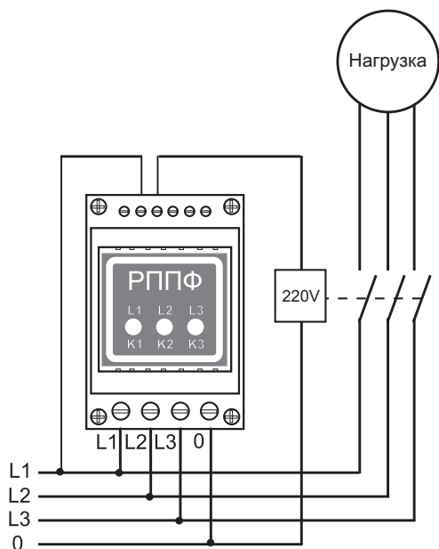
Рис.1 Вариант схемы подключения без контроля контактов пускателя.
