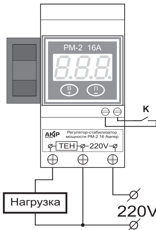
Рис. 1. Схема монтажа прибора.
