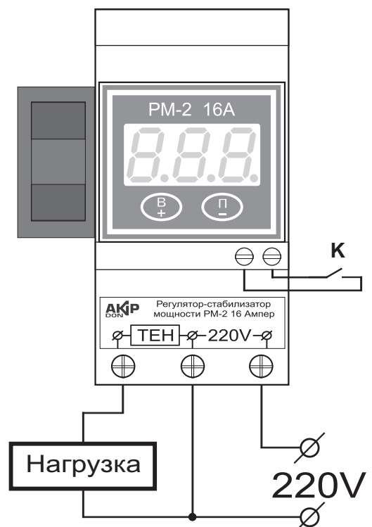
Рис. 1. Схема монтажа прибора.
