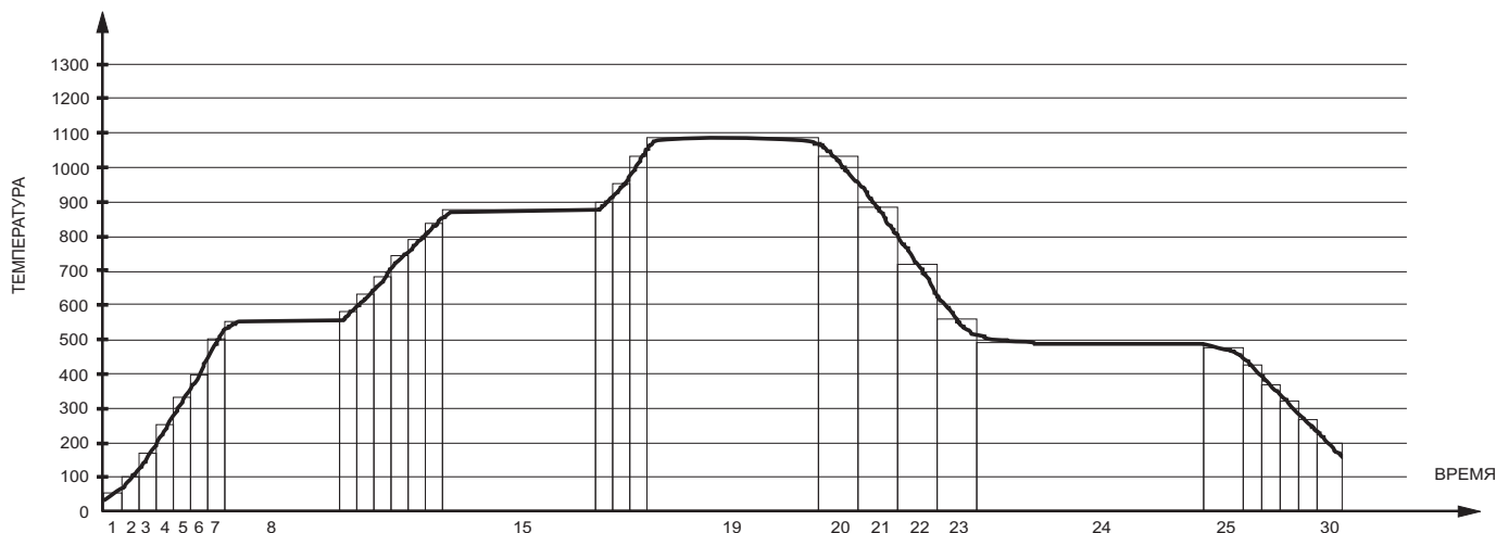
Рис.2 Условная схема профиля техпроцесса на 30 заданий (позиций) температура-время.
