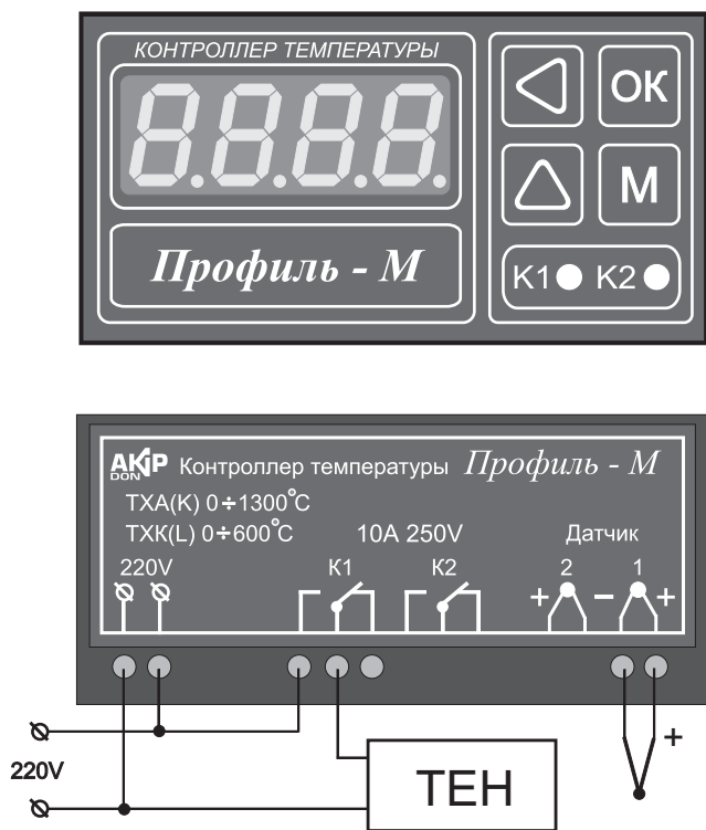
Рис. 1. Монтажная схема системы. Применяется при условии что мощность нагревательного элемента не превышает 1,5 киловатта.
