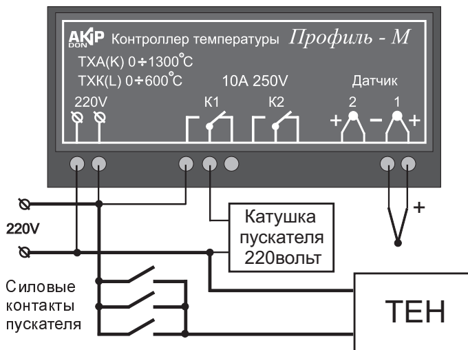
Рис. 2. Монтажная схема системы. Применяется при условии что мощность нагревательного элемента превышает 1,5 киловатта. Тип пускателя определяется мощностью нагрузки (ТЕНов).
