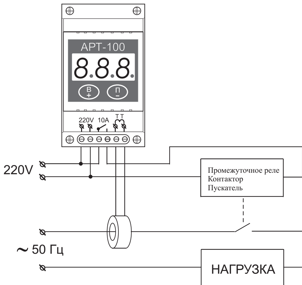
Рис.1 Вариант подключения прибора.
